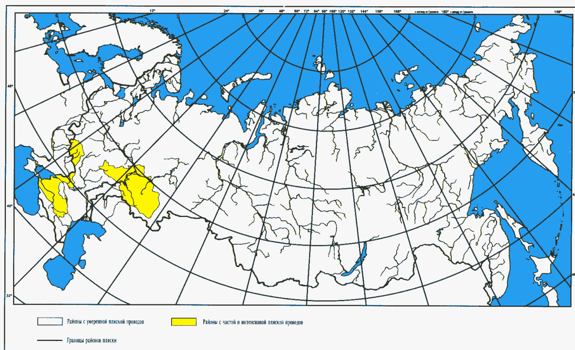
Рис. 2.5.4. Карта районирования территории РФ по пляске проводов
